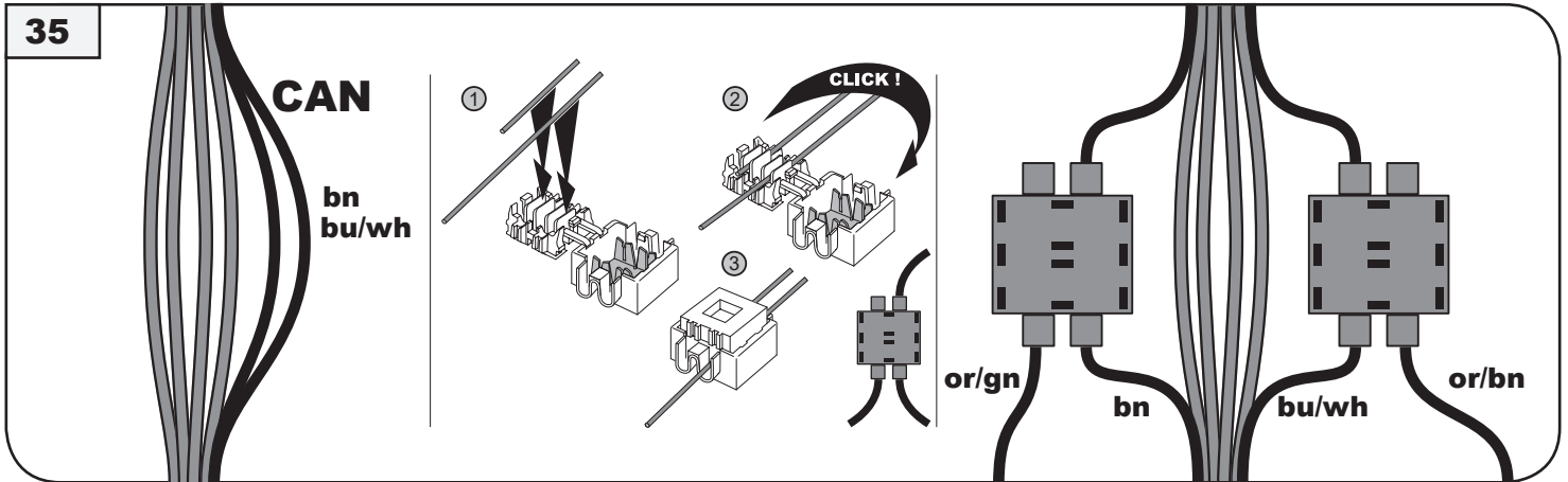
E-Satz or/gn → kabel bn, E-Satz or/bn → kabel bu/wh e-kit or/gn → kabel car bn, e-kit or/bn → kabel car bu/wh
